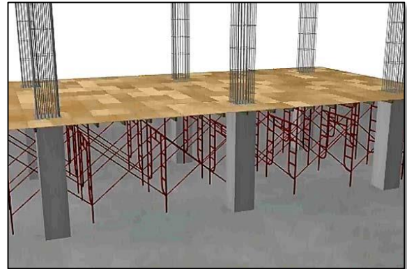
شکل ۱۳: مراحل اجرای سقف پس کشیده به روش غیر چسبنده
